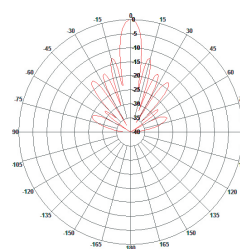
H-Plane Pattern
